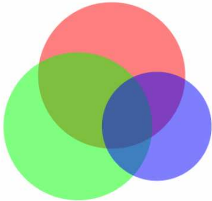
All genes
