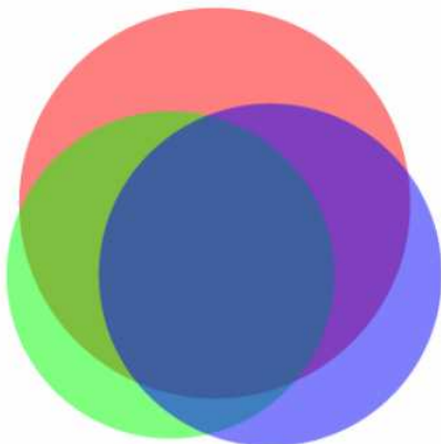
PC 2
