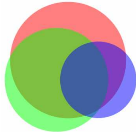
PC 4
