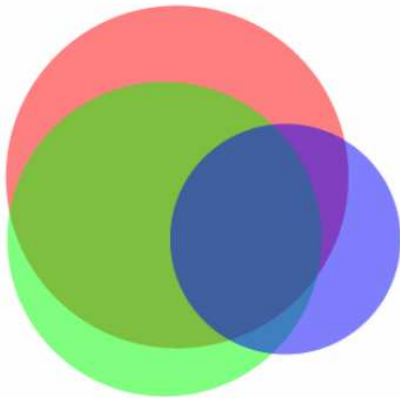
PC 1
