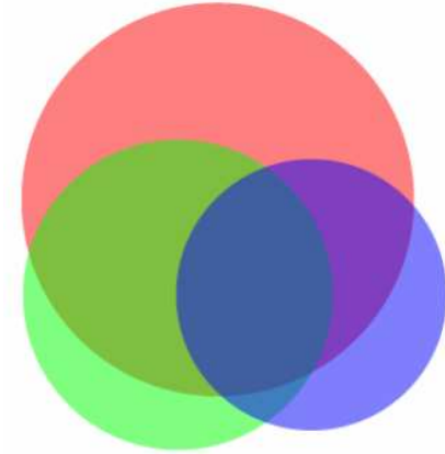
PC 3
