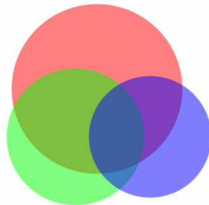
PC 5
